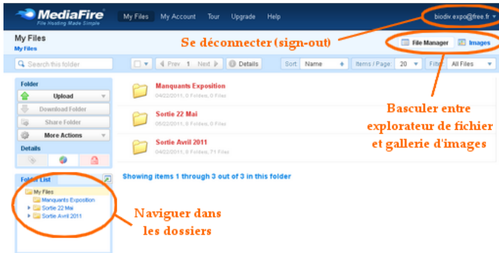
Figure 3 – Fenêtre principale – Aspect et principales zones d'interaction. Le site est organisé comme une arborescence dont la racine s'appelle 'My Files'.
